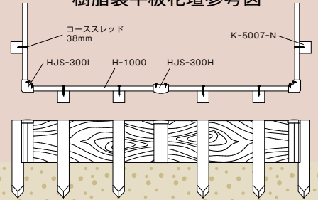
樹脂製平板花壇参考図
